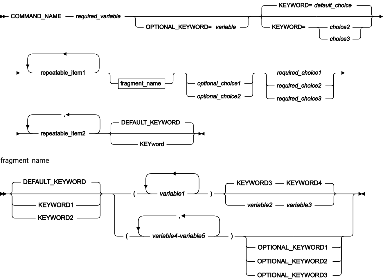
図 1. Syntax
