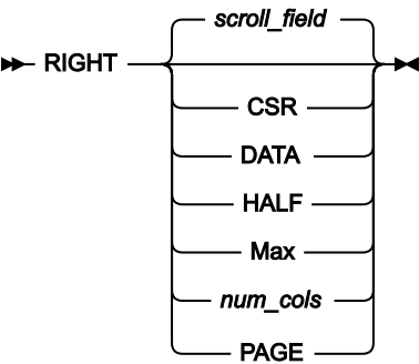
図 170. Template editing
