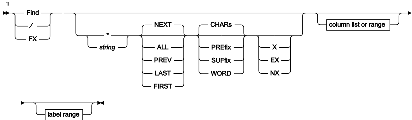
図 149. Editor session
