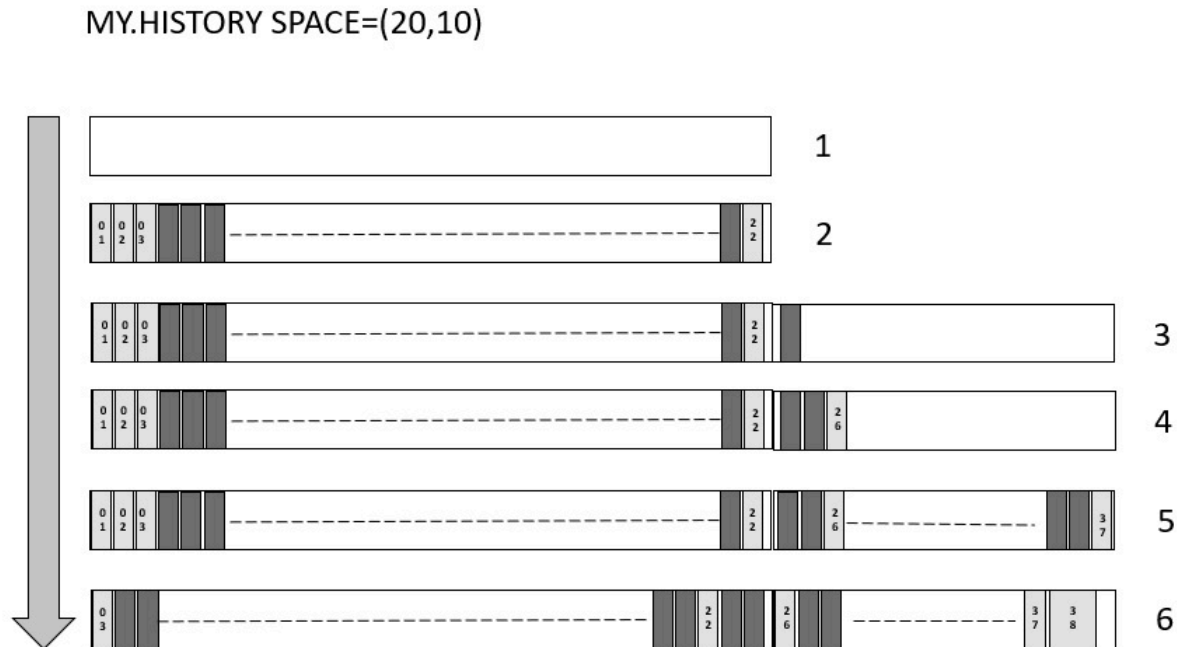
図 188. AUTO で管理される PDSE 履歴・ファイルの例
