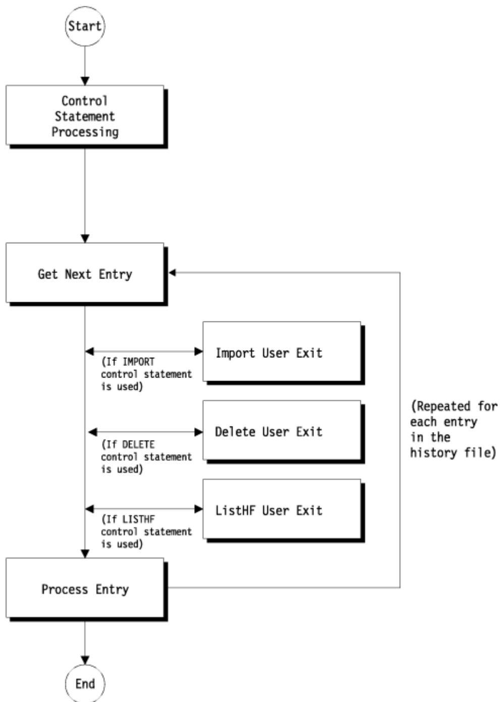
図 226. IDIUTIL バッチ・ユーティリティー出口点
