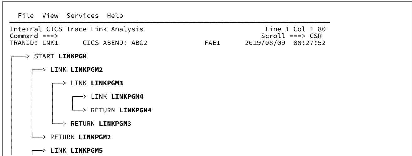
図 108. サンプル「CICS Trace Link Analysis」画面
