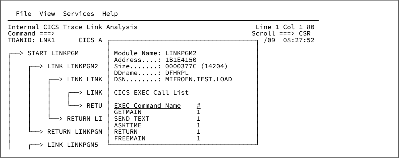
図 109. サンプル「CICS Trace Link Analysis」追加情報画面
