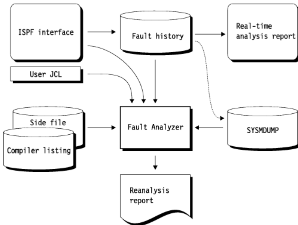
図 5. 再分析
