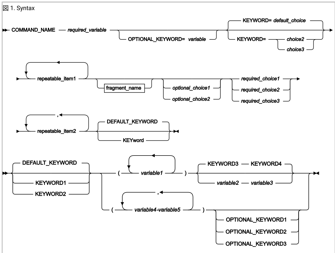
図 1. 構文図の例
