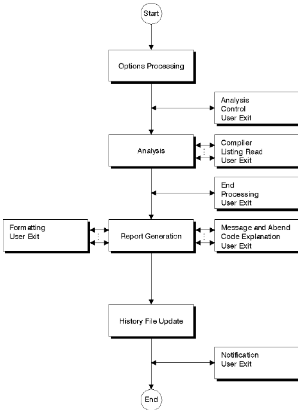
図 225. Fault Analyzer 分析の出口点 (IDIDA)
