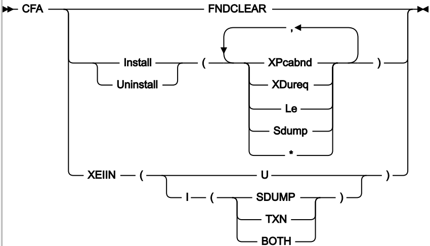
図 207. CFA command syntax
