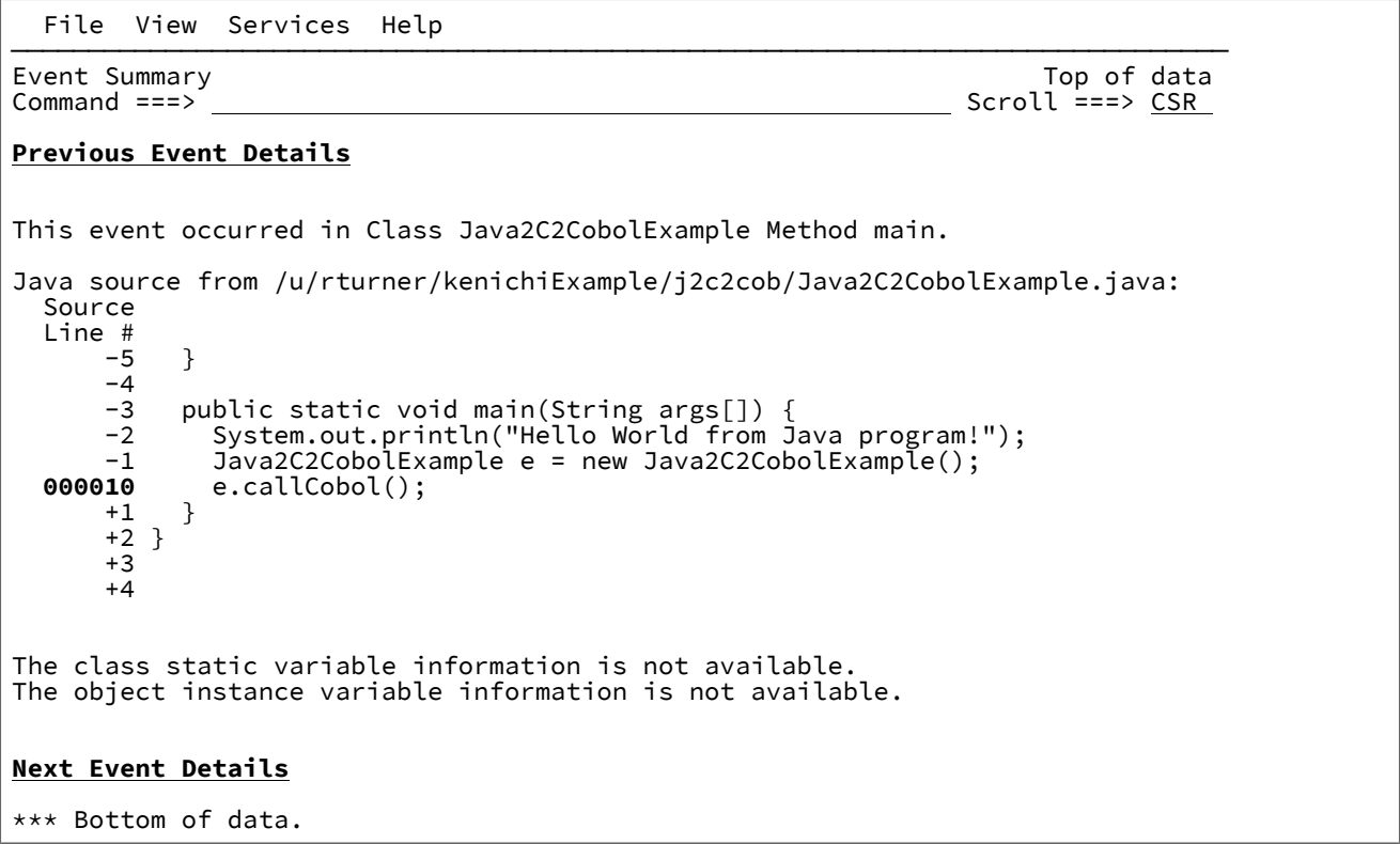
図 180. Java Event Details 画面の例
