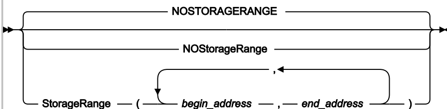
図 337. Syntax
