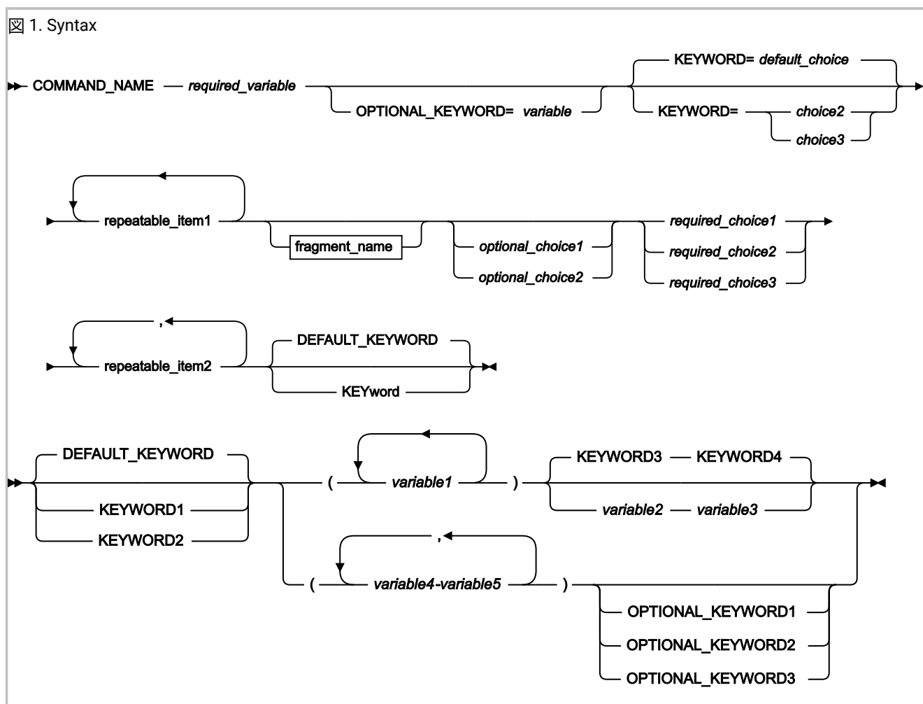
図 1. 構文図の例
