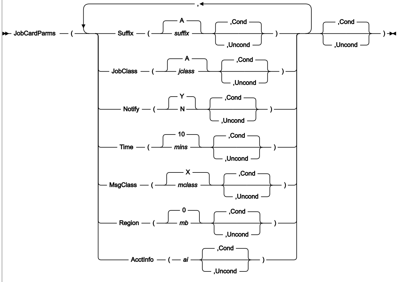
図 305. Syntax
