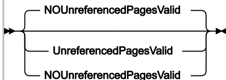
図 339. Syntax
