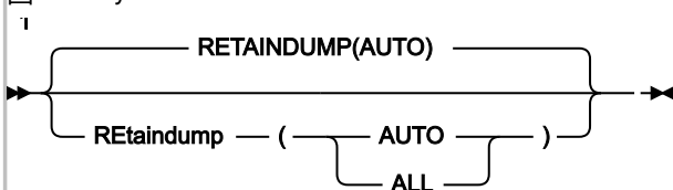
図 332. Syntax
