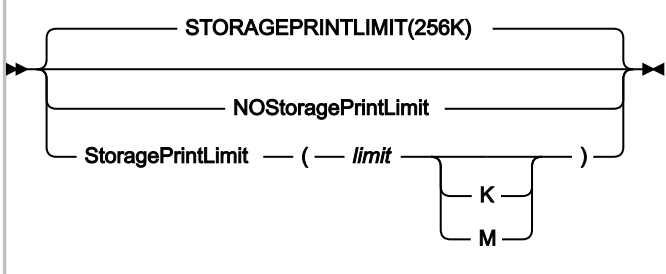
図 336. Syntax
