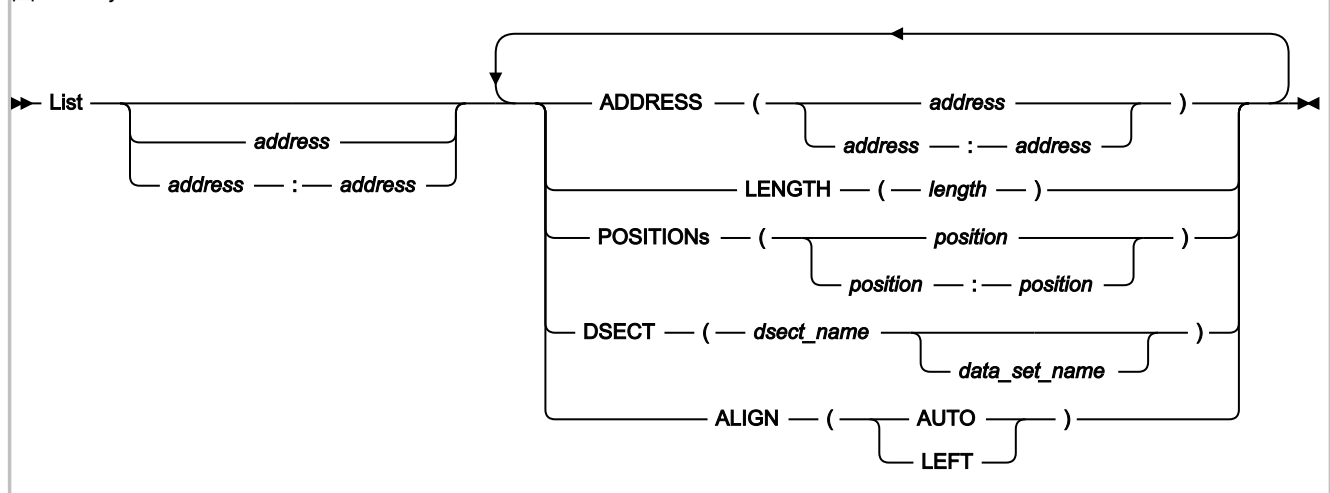
図 265. Syntax
