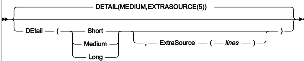
図 295. Syntax
