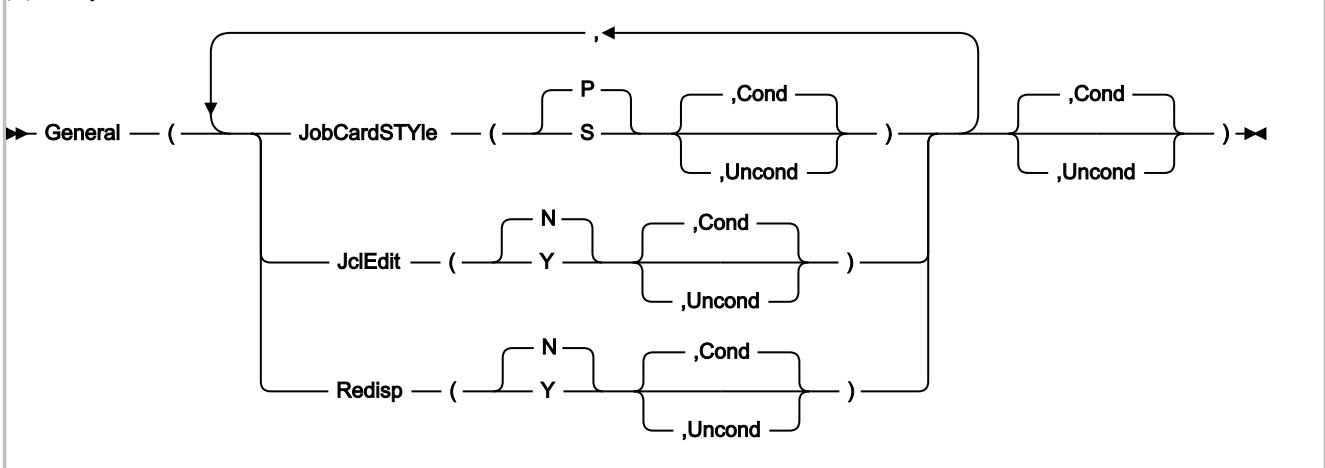
図 63. Syntax
