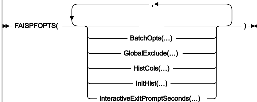
図 302. Syntax
