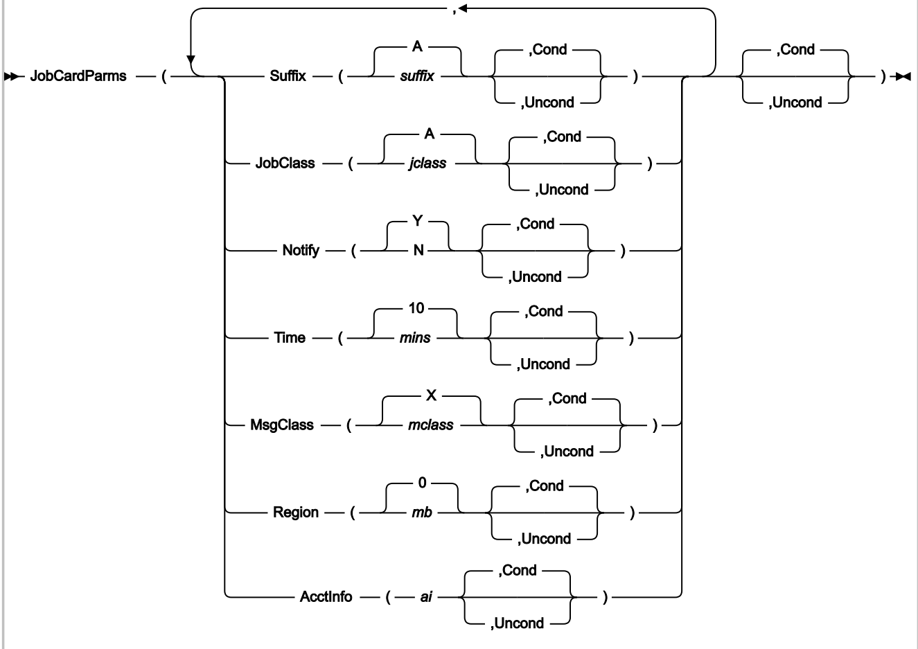
図 64. Syntax
