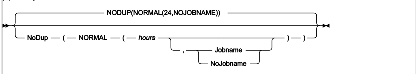
図 323. Syntax
