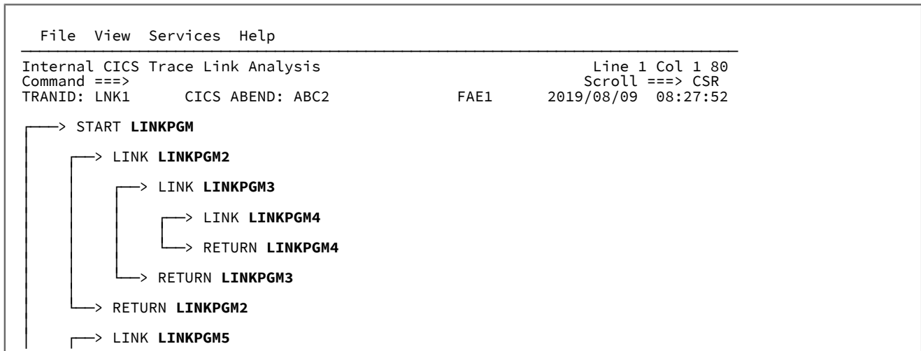
図 109. サンプル 「CICS Trace Link Analysis」 画面
