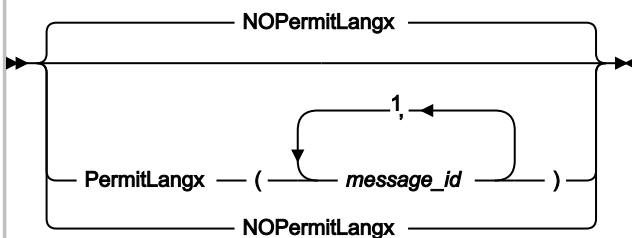
図 326. Syntax
