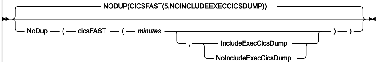
図 321. Syntax
