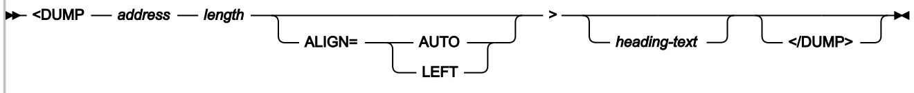
図 277. Syntax
