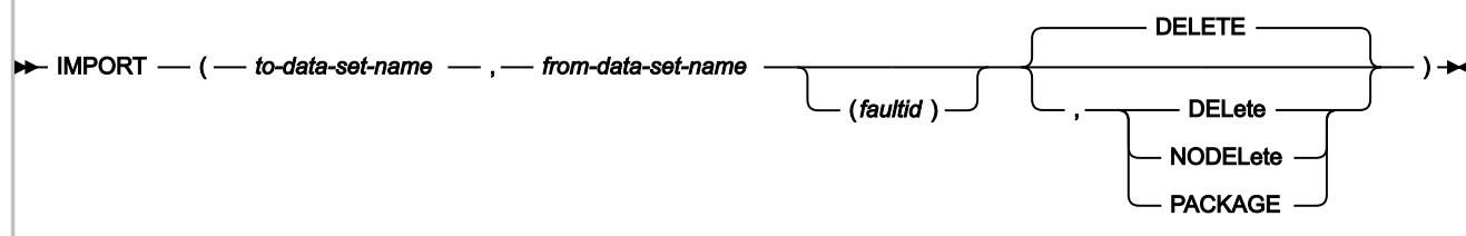
図 217. Syntax
