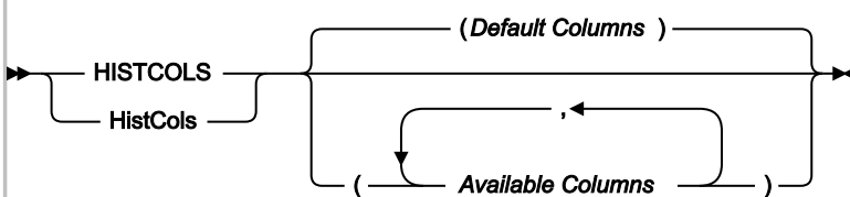
図 308. Syntax
