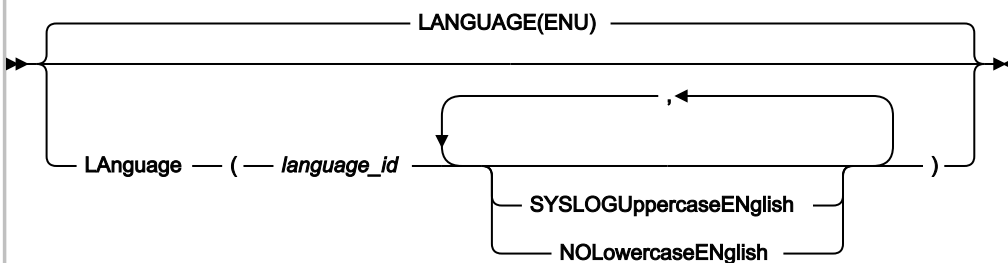
図 314. Syntax
