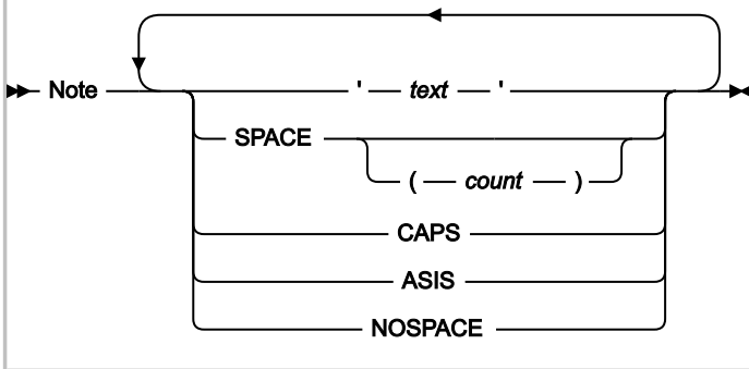
図 267. Syntax
