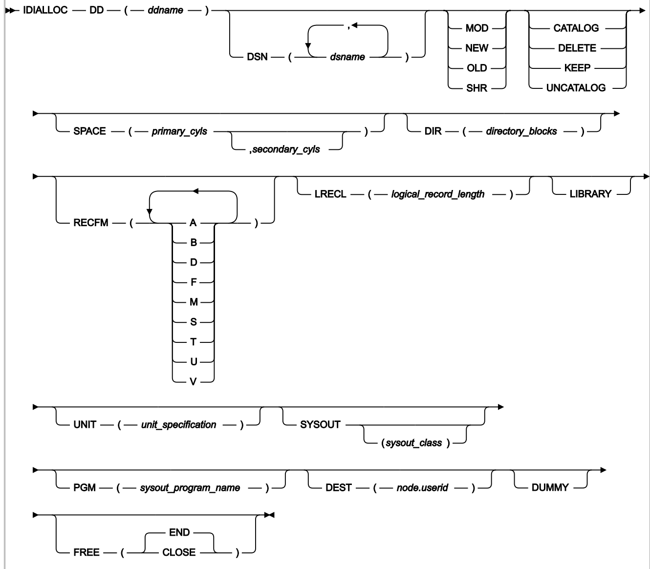
図 243. Syntax
