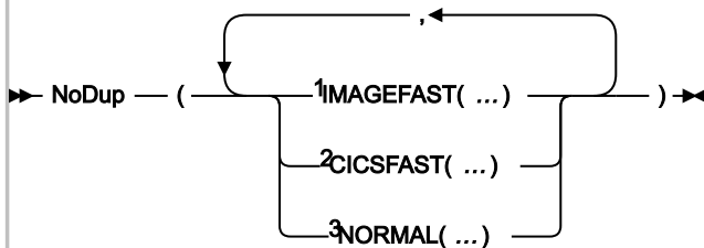
図 319. Syntax
