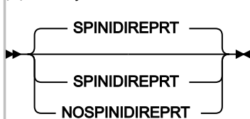
図 335. Syntax
