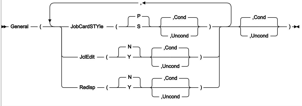
図 304. Syntax
