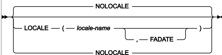
図 316. Syntax
