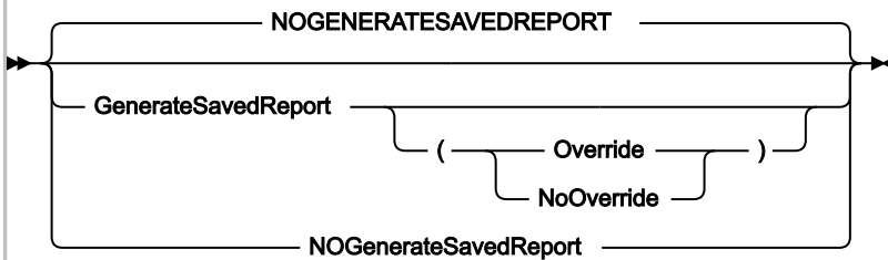
図 312. Syntax
