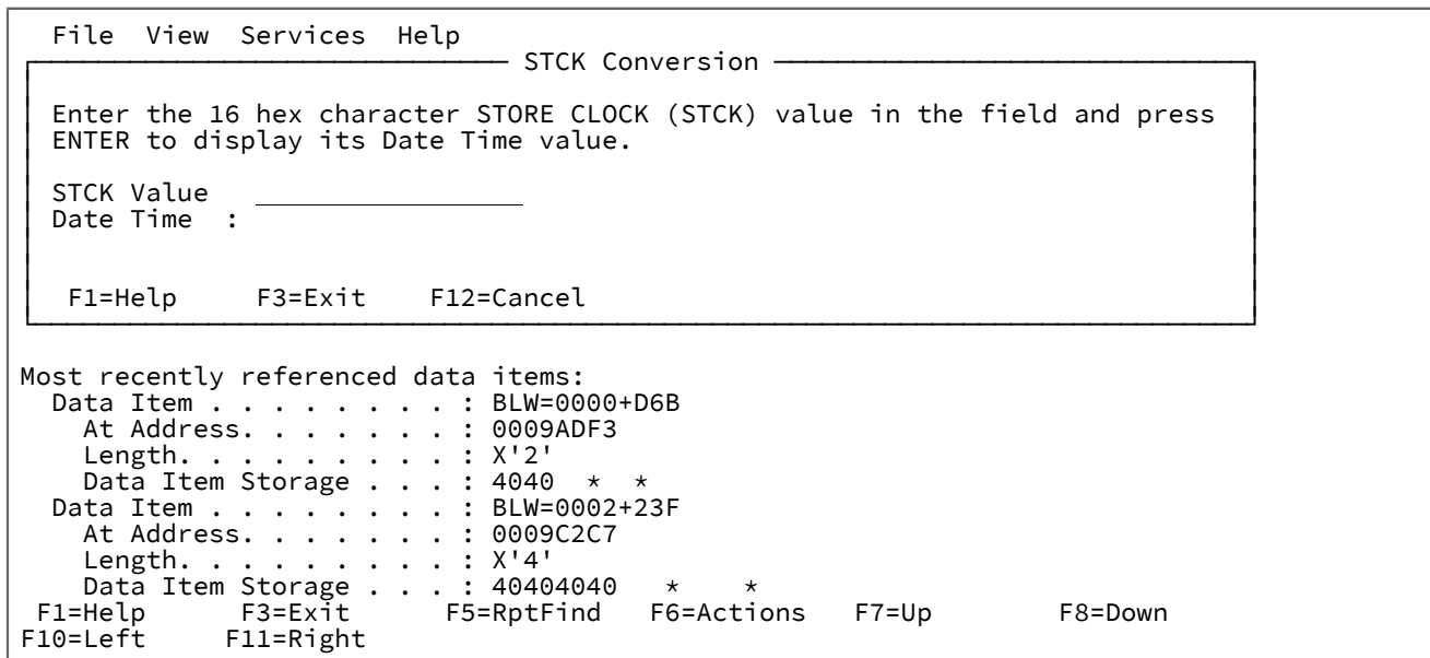
図 154. STCK Conversion 画面の例
